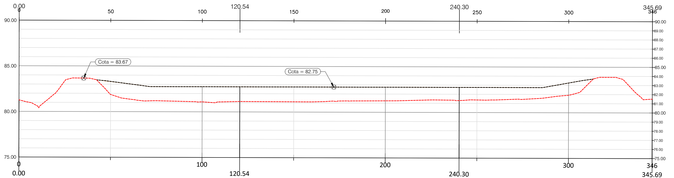
Perfil Long: 0+000.00 - 0+345.69 Rel Escala: Hor/Vert= 1/5
