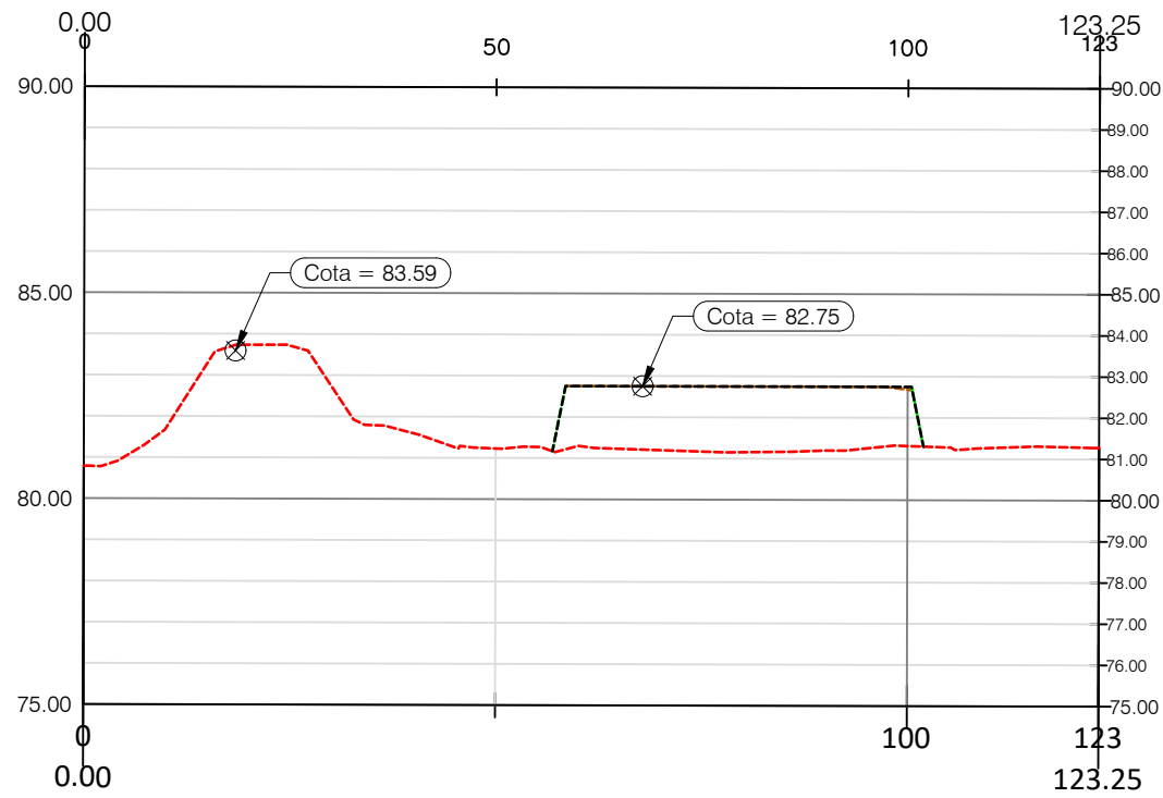
Perfil 1-1: 0+000.00 - 0+123.25 Rel Escala: Hor/Vert= 1/5
