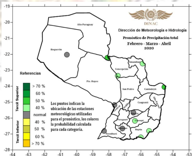
Figura 4. Pronóstico de Precipitación trimestre FMA 2020.
